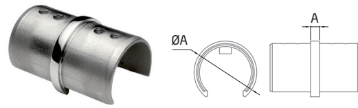
CT-212 AISI-304
