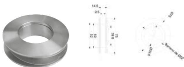
Jaladera hueca para puertas corredizas • Material: Acero inoxidable. • Acabado: Satín.
