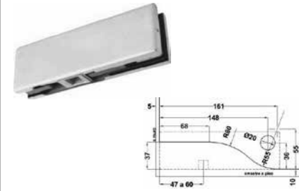
Herraje inferior para bisagra hidráulica. Acabado: Satín y cromo.
