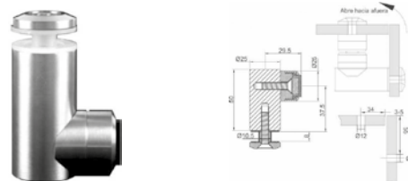
Tope para puerta con imán. Fijación al vidrio. Se necesita perforación de 12 mm. • Material: Acero inoxidable.
