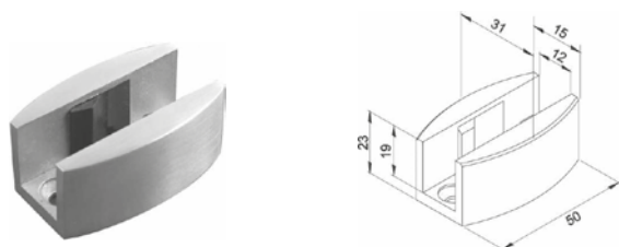
Guía de piso para puerta corrediza. Fijación a piso. • Material: Acero inoxidable.
