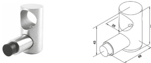
Tope lateral para sistema corredizo. Fijación en tubo. • Material: Acero inoxidable.
