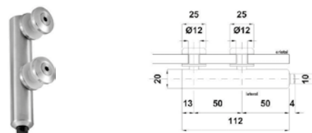
Tope vidrio - vidrio con fijación a vidrio. El vidrio requiere perforación para su fijación. • Material: Acero inoxidable. • Acabado: Satín.
