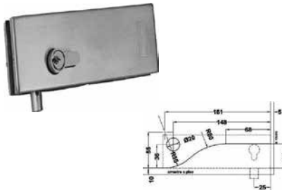
Chapa a piso con resaque. Acabado: Satín y cromo.
