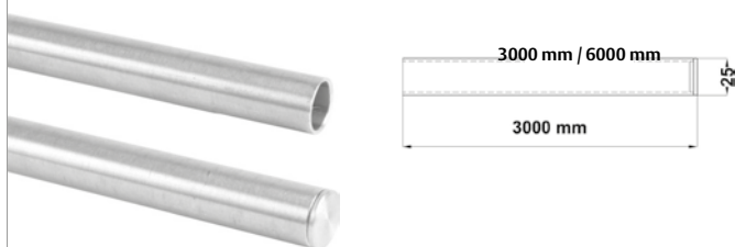
Tubo para sistema corredizo y 1" de diámetro Cal. 18. • Material: Acero inoxidable. • Medidas: 3 m y 6 m de longitud.
