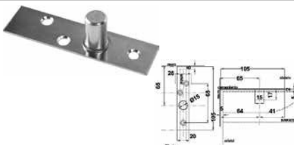
Punto de giro para herraje superior.
