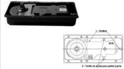
Bisagra hidráulica para 80 Kg. Medidas para perforación a piso: 100 x 266 x 51 mm.
