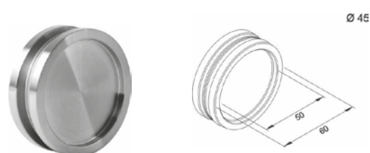
Jaladera para puerta de vidrio templado en sistema corredizo. Se necesita perforación de 15 mm. • Material: Acero inoxidable.
