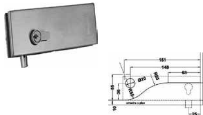
Chapa a piso con resaque. Acabado: Satín y cromo.
