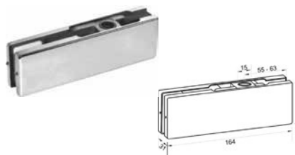
Herraje superior para punto de giro superior. Acabado: Satín y cromo.
