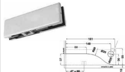
Herraje inferior para bisagra hidráulica. Acabado: Satín y cromo.
